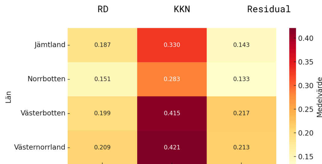
Figur 7. Heatmap som visar medelvärde för RD, KKN och residual på regional nivå.
