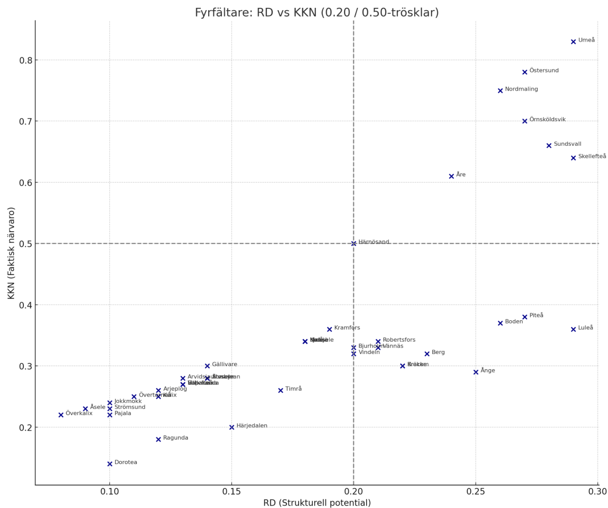
Figur 4. Fyrfältaren illustrerar position utifrån potential för och utfall av KKN.
