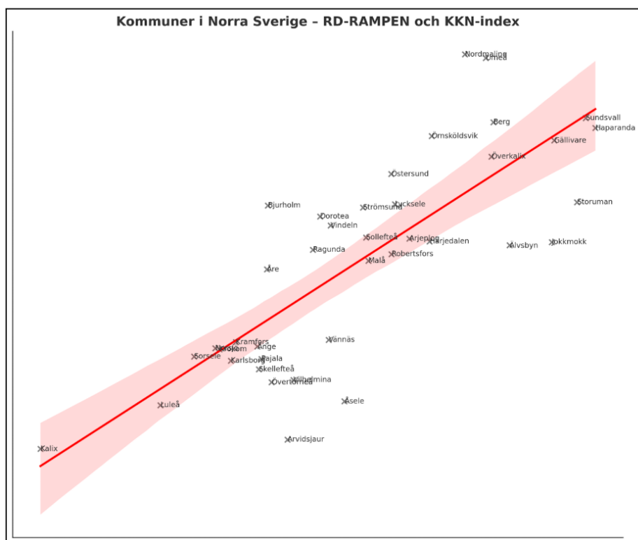
Figur 3. Korrelationen illustrerad i regressionslinjen visar att styrkan i det linjära sambandet är r = 0,79 . Förklaringsgraden formuleras 0,79^2 = 0,624 ( r^2 ) \rightarrow 62,4 % av variationen i KKN förklaras av RD-RAMPEN:KKN.
